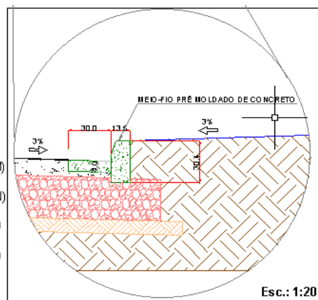
DETALHE ESTRUTURAL CONCRETO ARMADO - CA PAVIMENTO PARA TRÁFEGO MÉDIO N=1 x10 6
